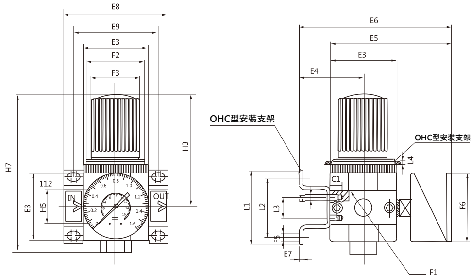
外形尺寸/Dimension
